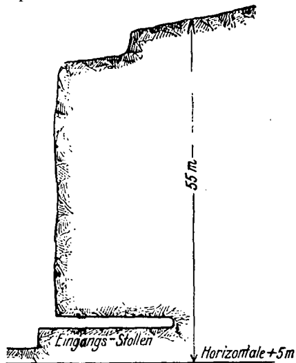
Schnitt durch den Eingangsstollen 1:250
